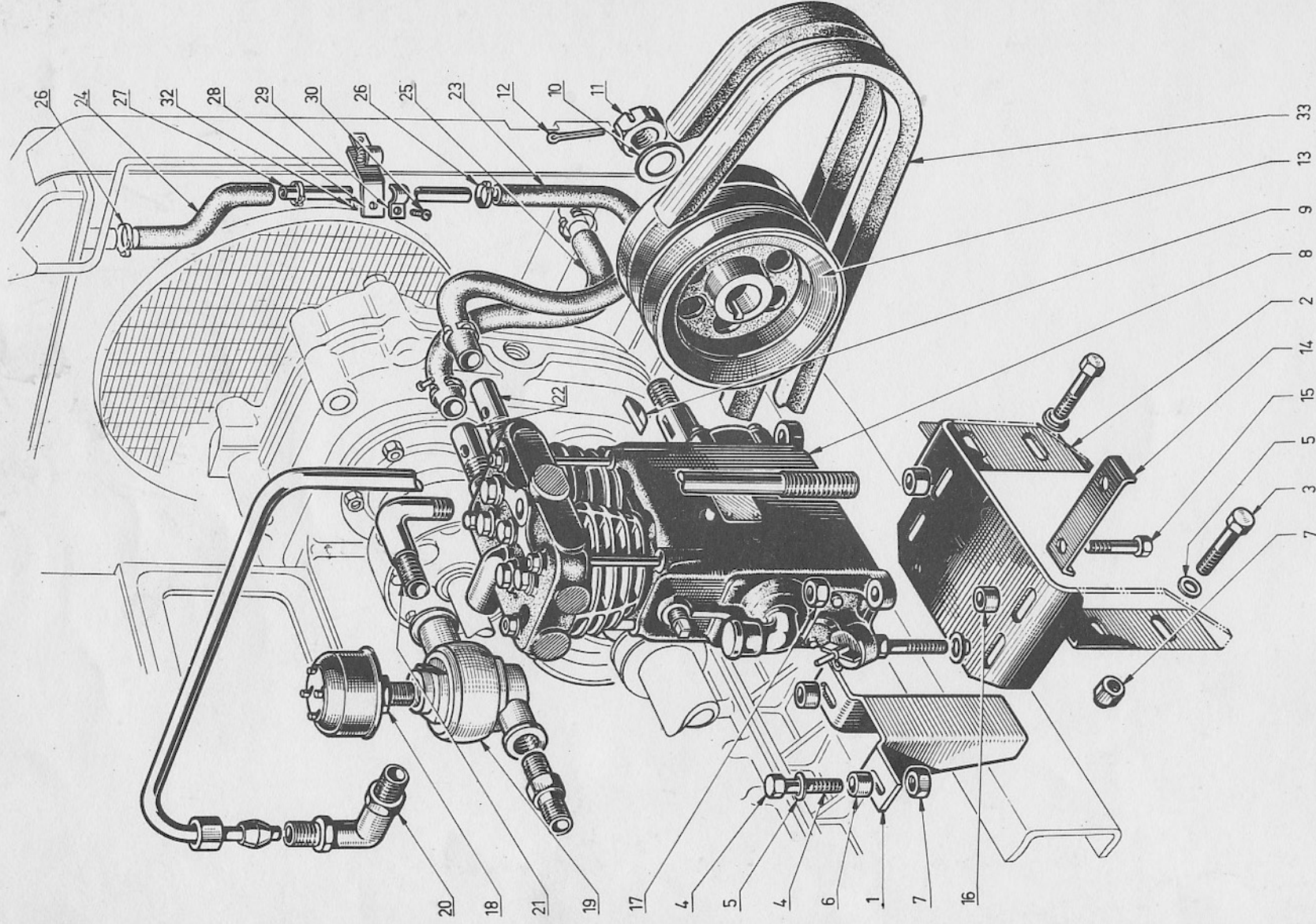
SG 67- INSTALLATION du COMPRESSEUR
