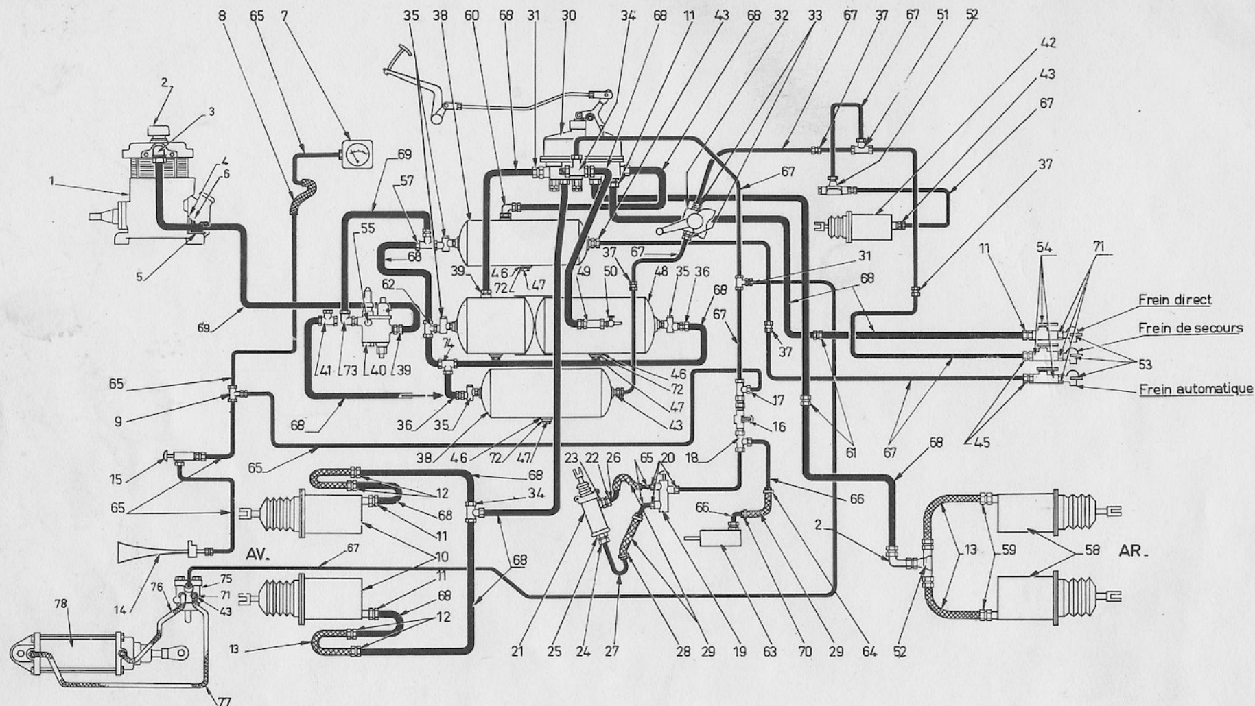
SG.66 NOUVELLE INSTALLATION d'AIR COMPRIMÉ sur CHASSIS ZU121 - ZU122.
