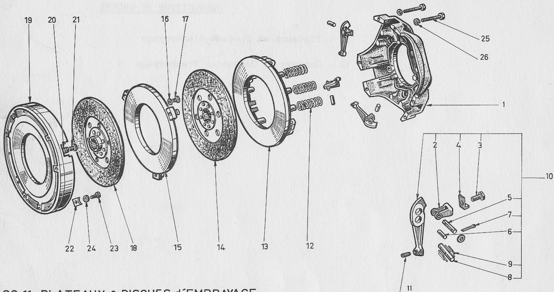
SG.11_PLATEAUX & DISQUES d'EMBAYAGE
