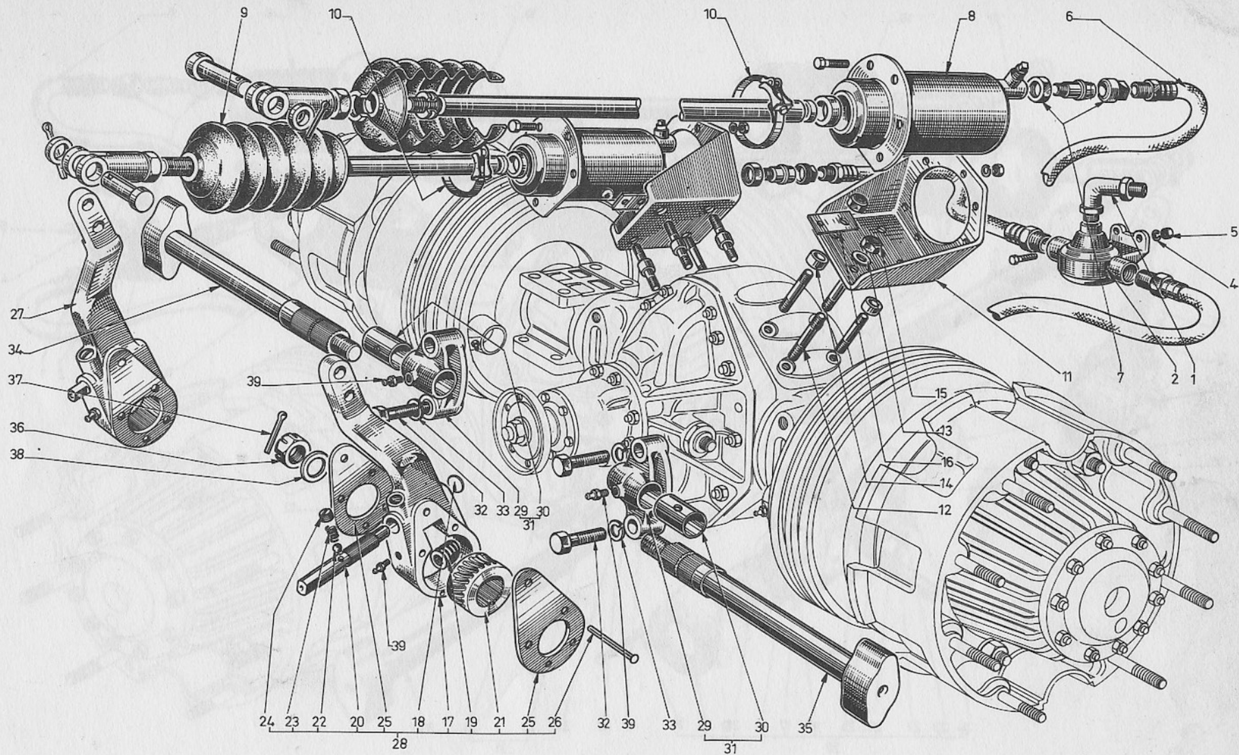
SG-62 COMMANDE DES FREINS ARRIERE (ZU 122)
