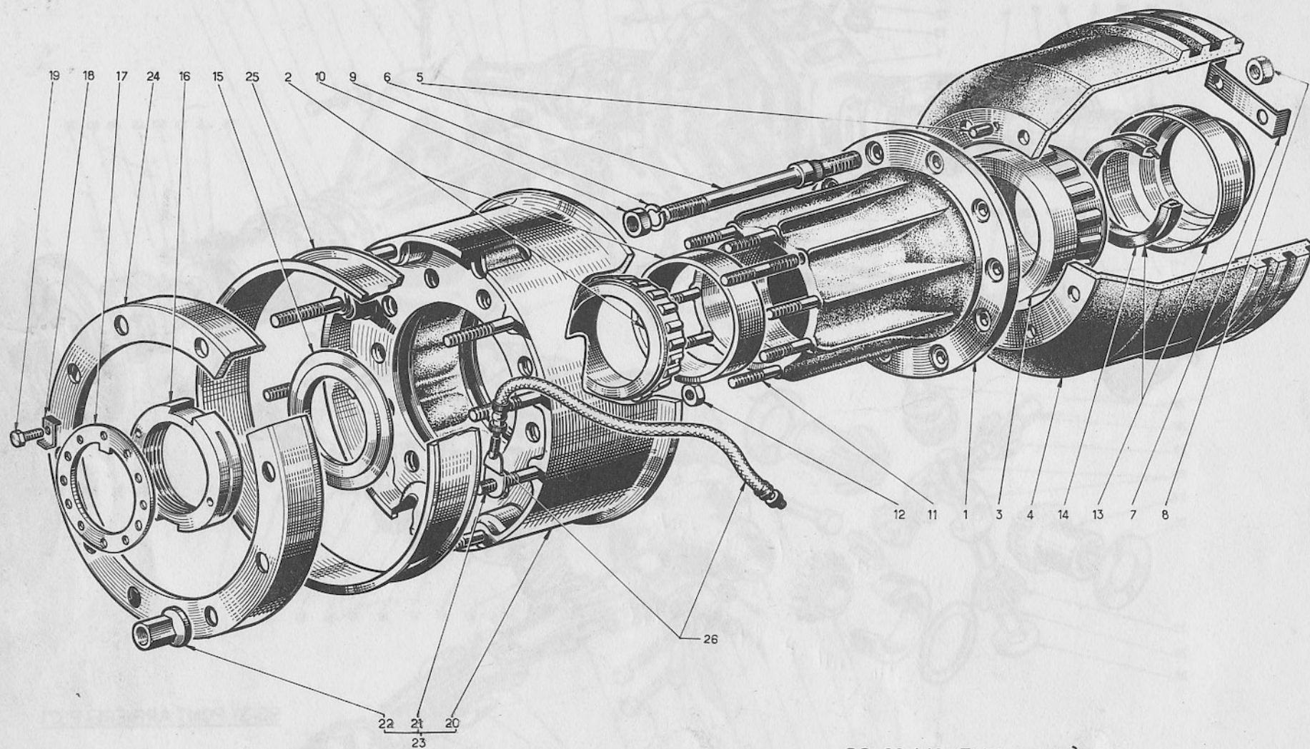
SG-32 MOYEUX ARRIÈRE
